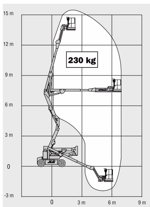
JLG E450AJ
